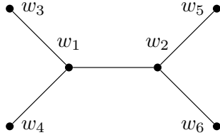
図 5: H グラフ \Gamma
