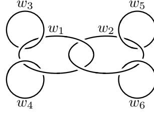
図 6: 手術図式 \mathcal{L}(\Gamma)
