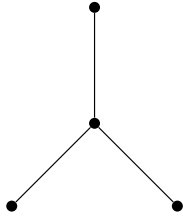
図 3: Brieskorn 多様体
