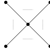
図 4: 手術図式に対応するグラフ
