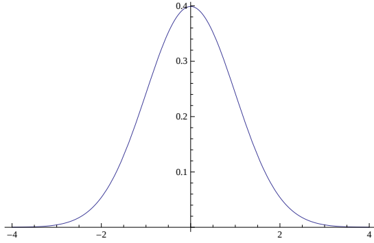
図 1: ガウス分布の確率密度関数
