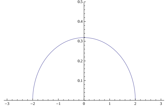
図 2: Wigner の半円分布の確率密度関数
