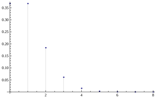
図 3: ポアソン分布 p_1
