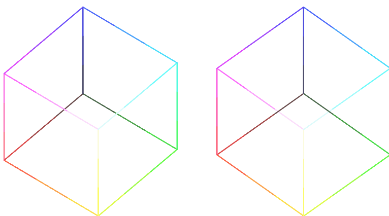
Figure 2: 正六面体
