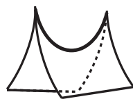
cuspidal edge
